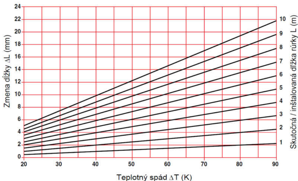
Diagram tepelnej rozťažnosti HERZ - PIPEFIX Plasthliníkovej rúrky PE-RT
